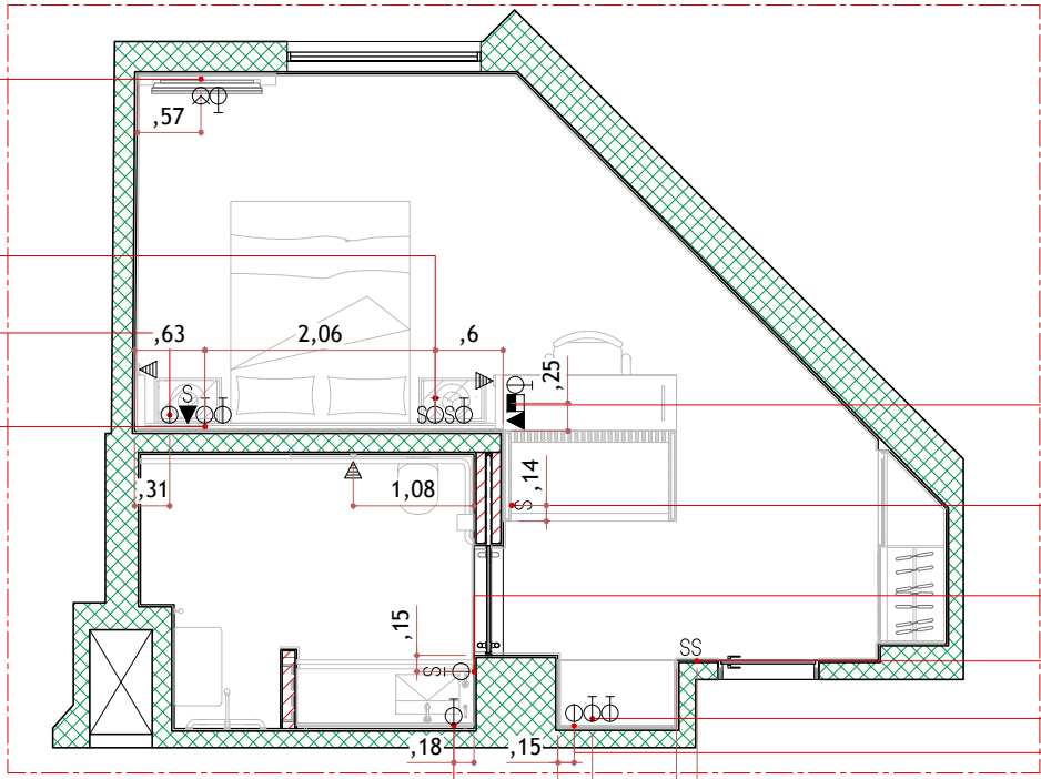
Planta - Pontos de elétrica Planta 6º ao 13º pavimento - esc. 1:75
