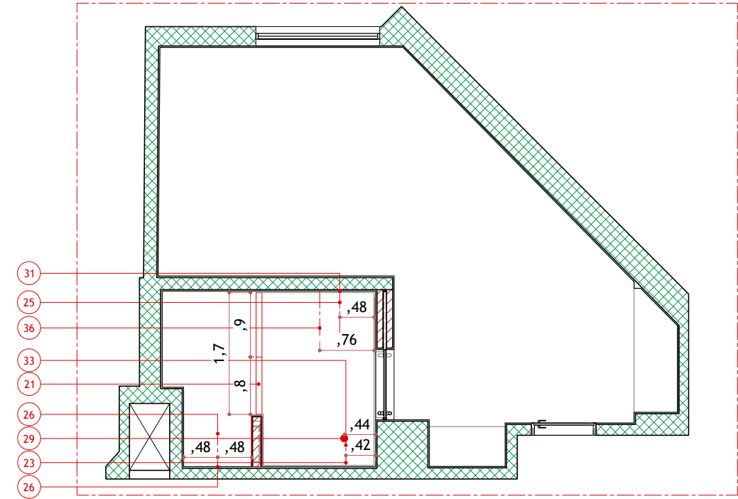
Planta - Eixos de hidráulica Planta 6º ao 13º pavimento - esc. 1:75
