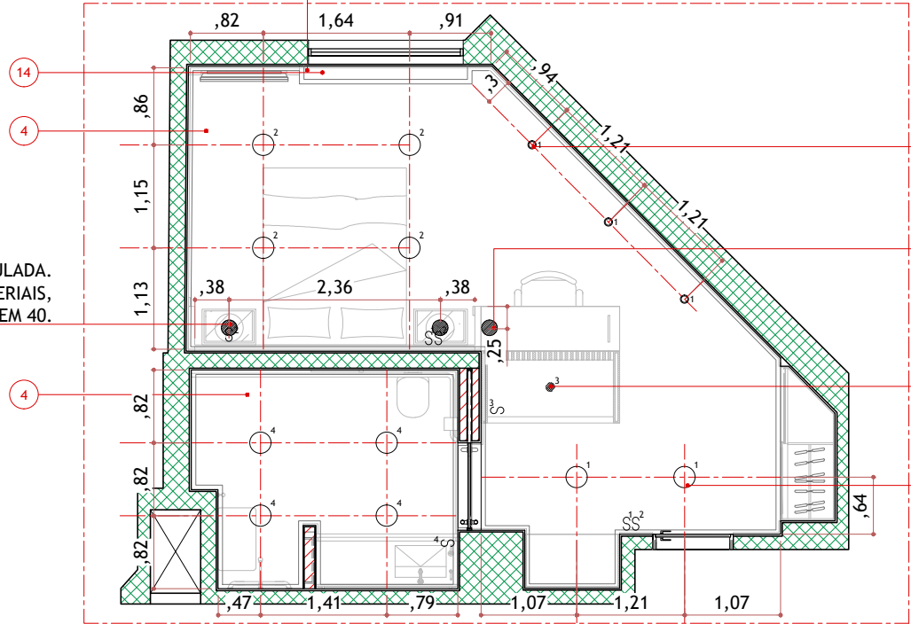
Planta - Forro e iluminação Planta 6º ao 13º pavimento - esc. 1:75
